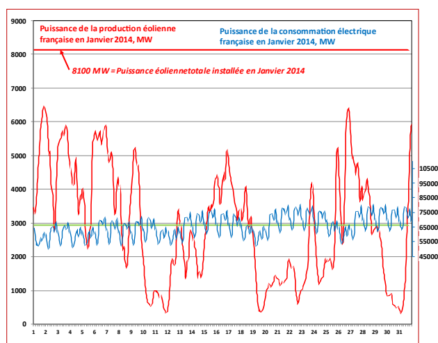
FIGURE 6 : PUISSANCE ÉOLIENNE ET CONSOMMATION D'ÉLECTRICITÉ EN FRANCE :
