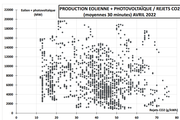
Figure 2. production d'éolien + solaire photovoltaïque et émissions de CO 2 de la production d'électricité française. D'après les données de RTE pour Avril 2022. Courtoisie Jean-Paul Hulot.
