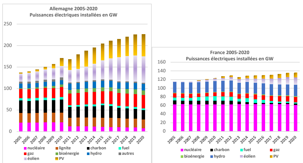
Figure 7 : évolution de 2005 à 2020 des puissances électriques installées, à gauche en Allemagne (données BMWE), à droite en France (courtoisie JP Riou). Les couleurs uniformes correspondent aux centrales pilotables, les couleurs en dégradé à l'éolien et au PV.
