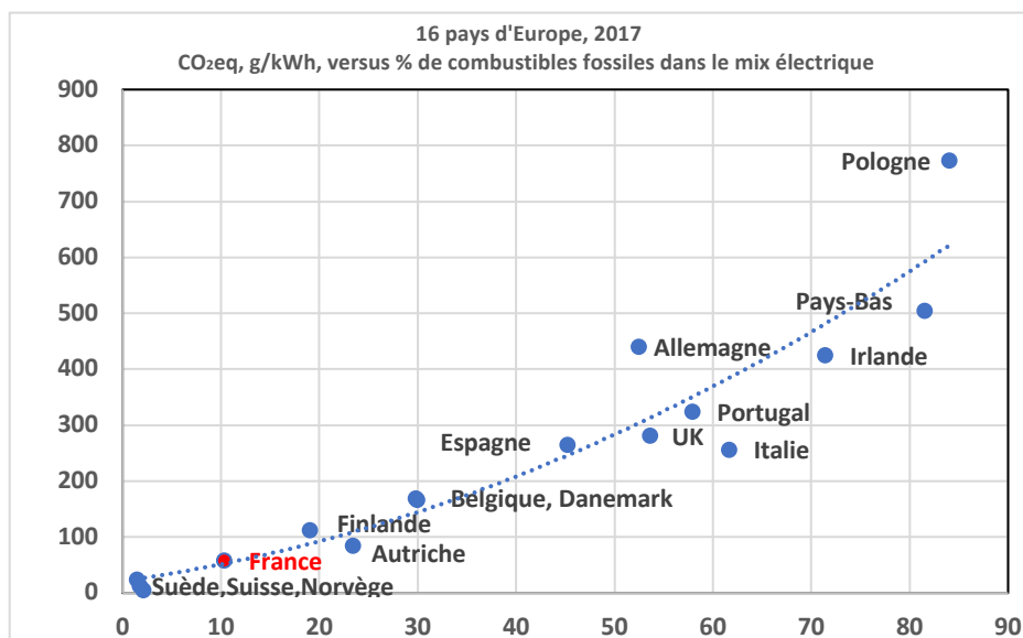
Figure 1: Emissions de CO 2 eq du mix de production électrique 2017 de 16 pays d'Europe de l'Ouest en fonction du % des combustibles fossiles dans ce mix. Les valeurs plus fortes d'émissions de CO 2 eq pour une même proportion de combustibles fossiles viennent essentiellement de la nature des combustibles utilisés, charbon plutôt que gaz. Source des données : Eurostat et Agence européenne de l'environnement.
