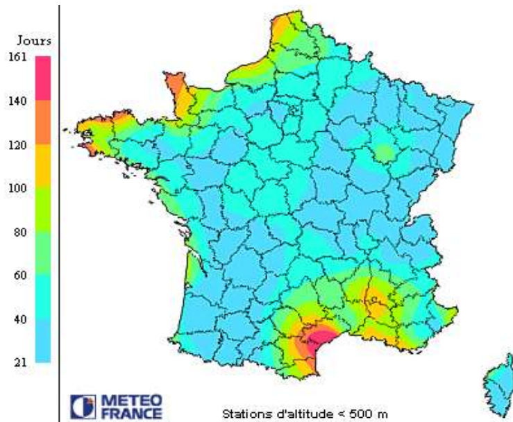
Carte des vents météo France
